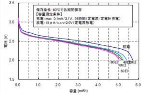
高温 (60°C) 保存特性
