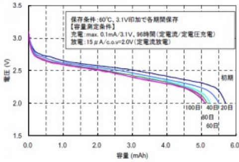
フロート充電特性 (60°C、3.1V印加)
