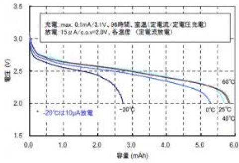
放電温度特性 (温度が及ぼす影響)
